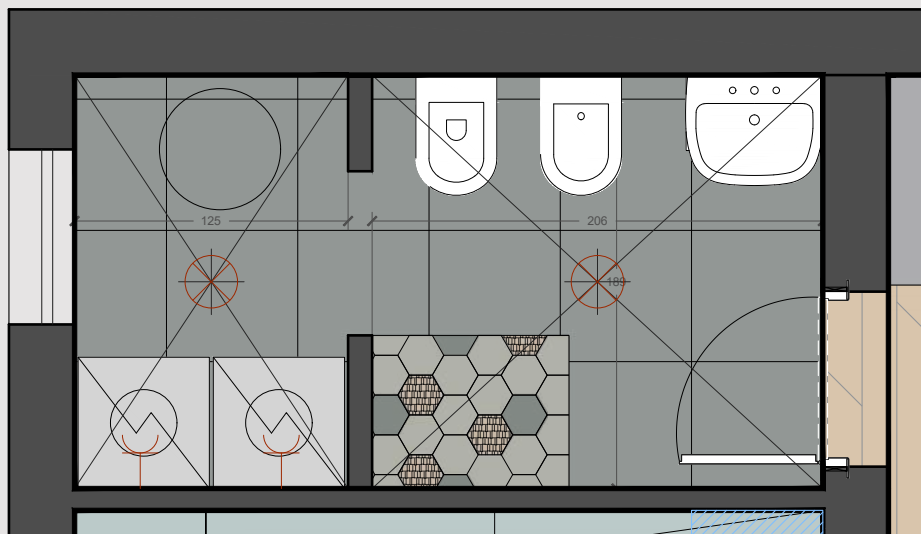
Es. Schema di posa dei pavimenti
