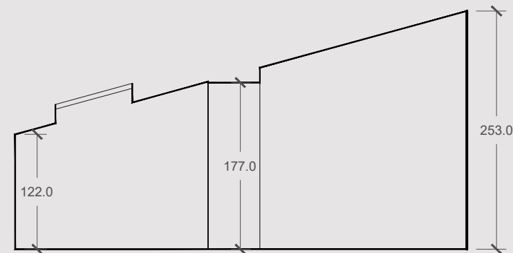
B Sezione
