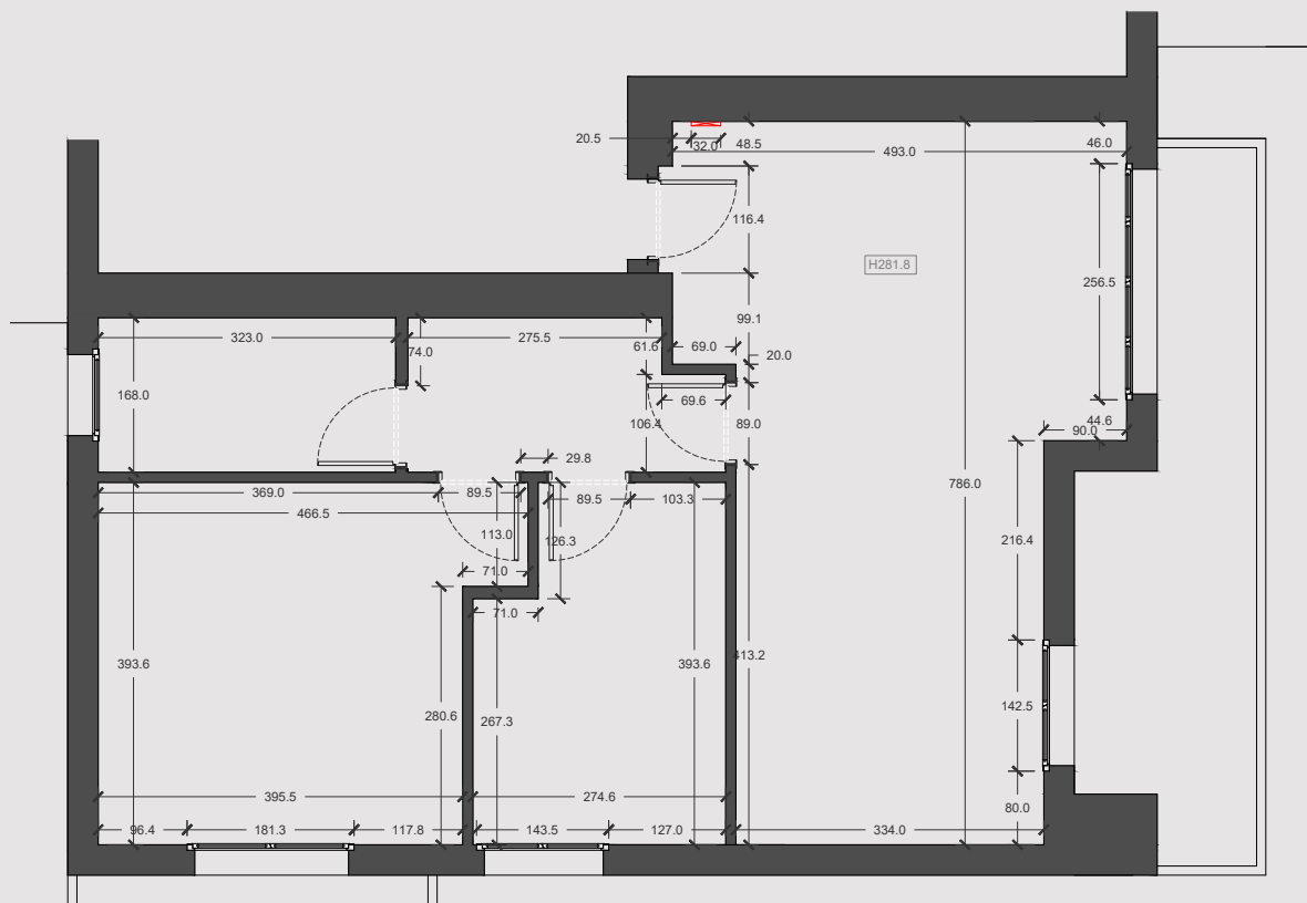
A Pianta
